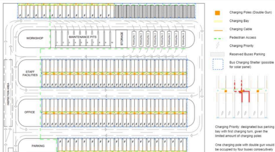
Gambar 37. Desain Depo Bus Listrik
