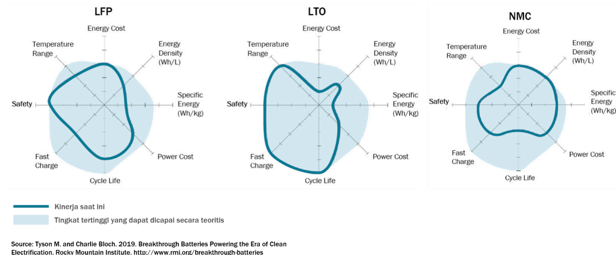
Gambar 7. Perbandingan Spesifikasi Teknologi Baterai
